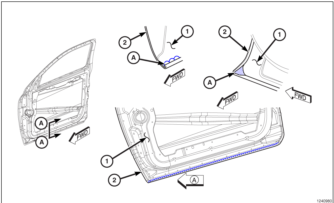
Fig. 59 Front Door – Standard Cab
