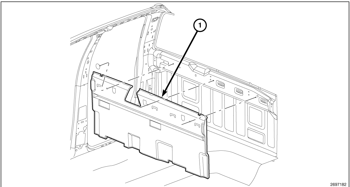
Fig. 42 CAB BACK
