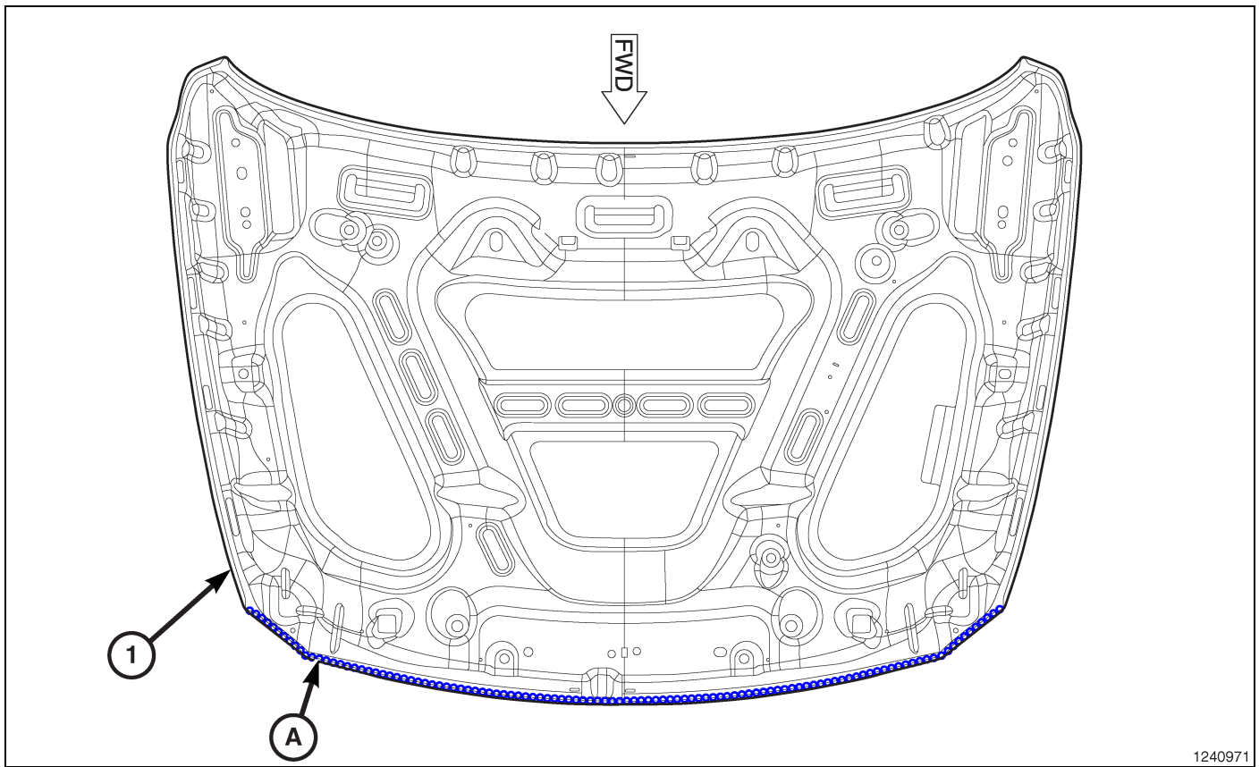
Fig. 58 Hood
