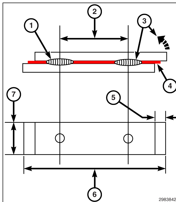
Fig. 23 Weld Coupon
