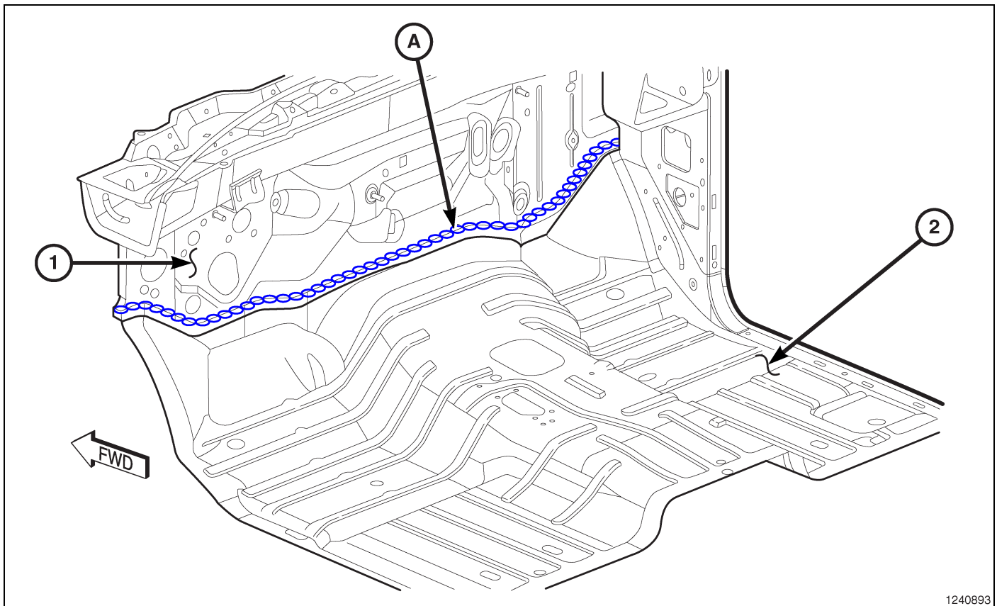
Fig. 51 Dash Panel/Front Floor Pan
