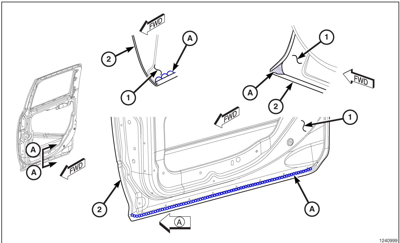
Fig. 61 Rear Door
