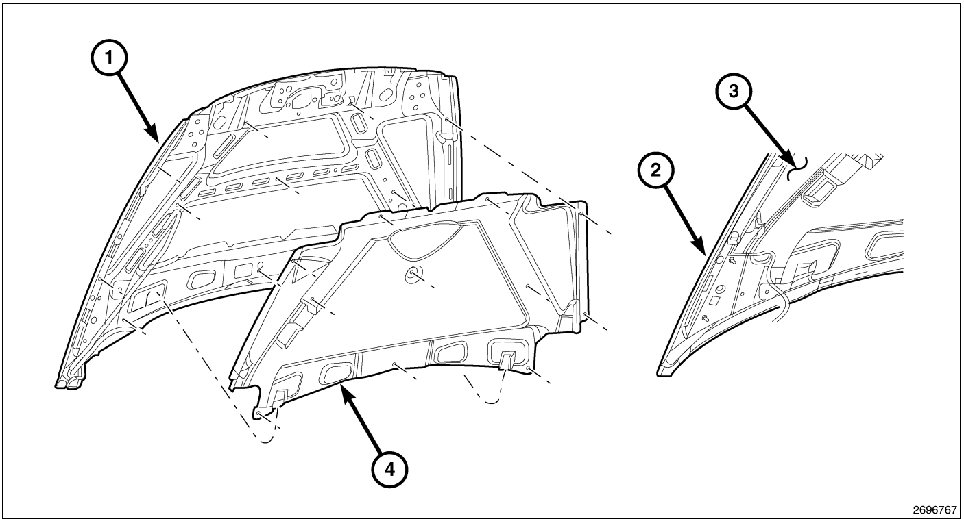
Fig. 31 HOOD
