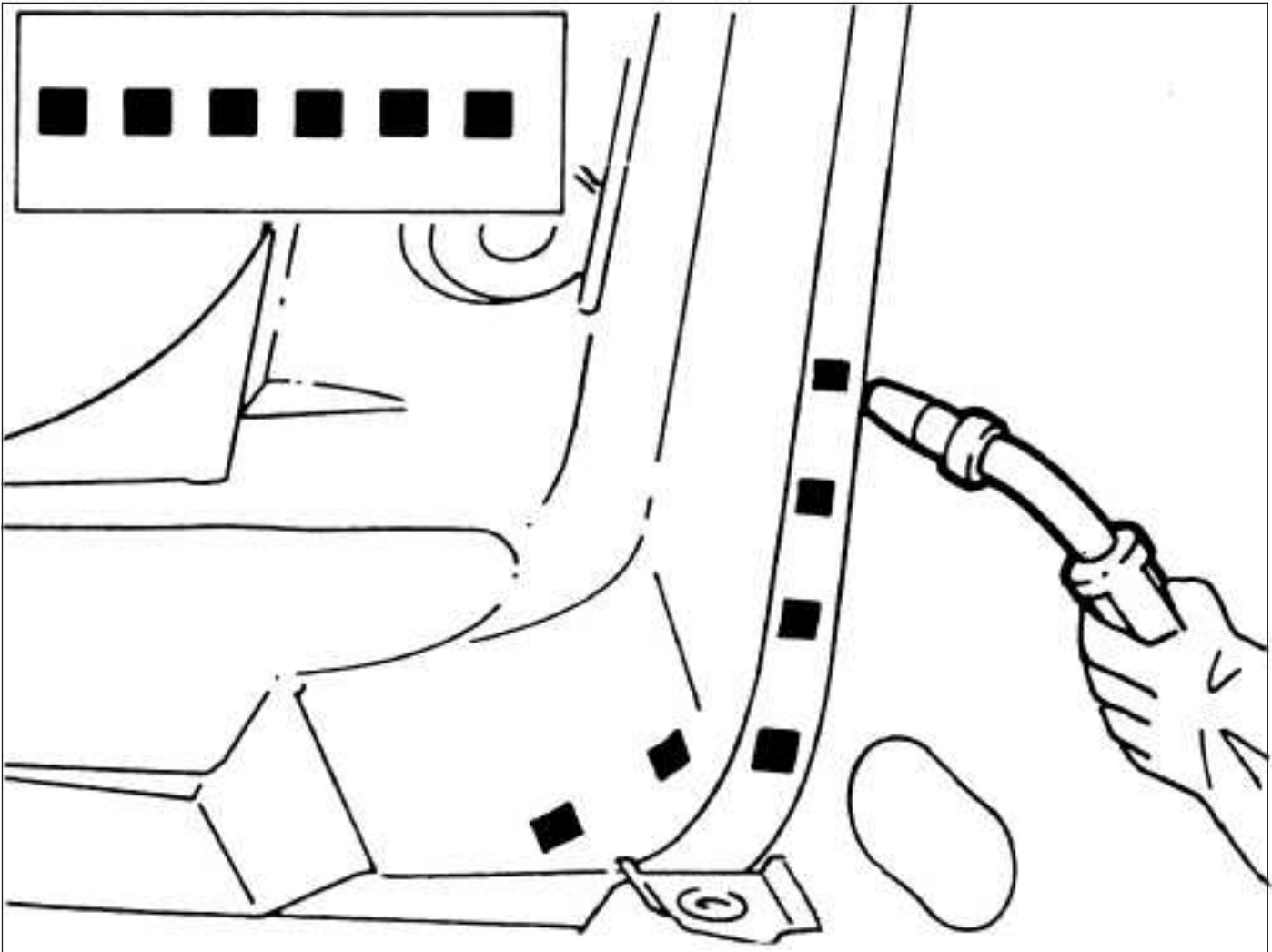
MIG fill/plug welding
