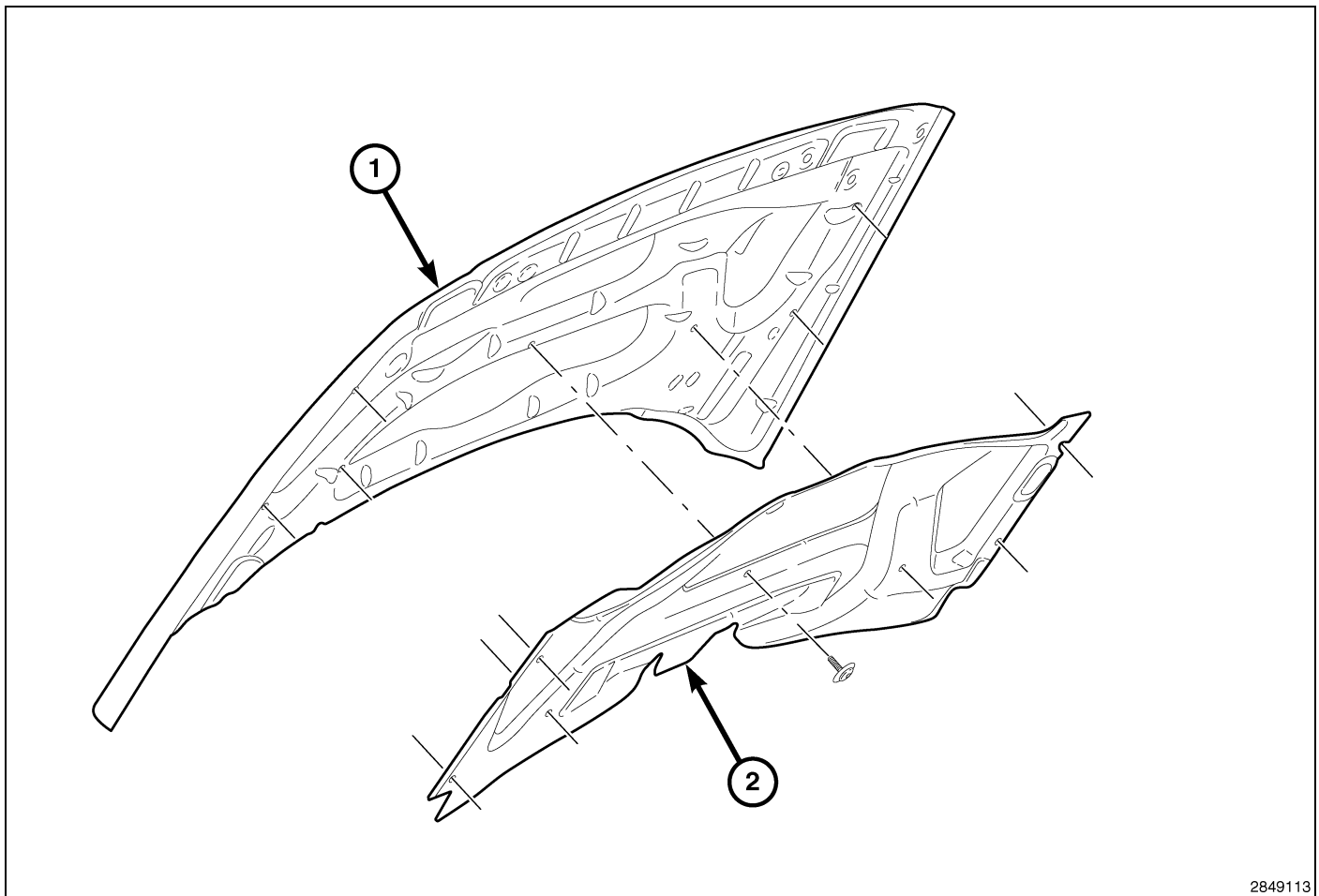
Fig. 29 Hood
