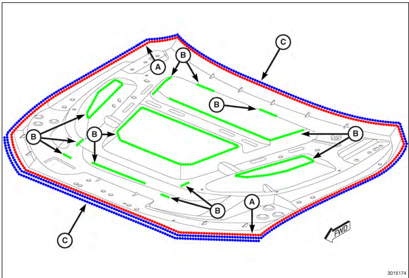
Fig. 49 Hood
