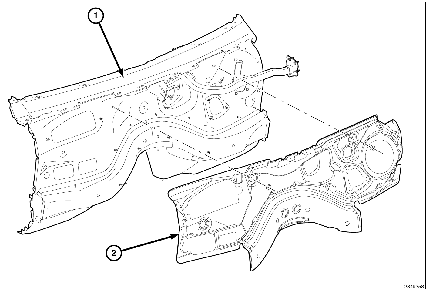
Fig. 33 Dash Panel (Outer)
