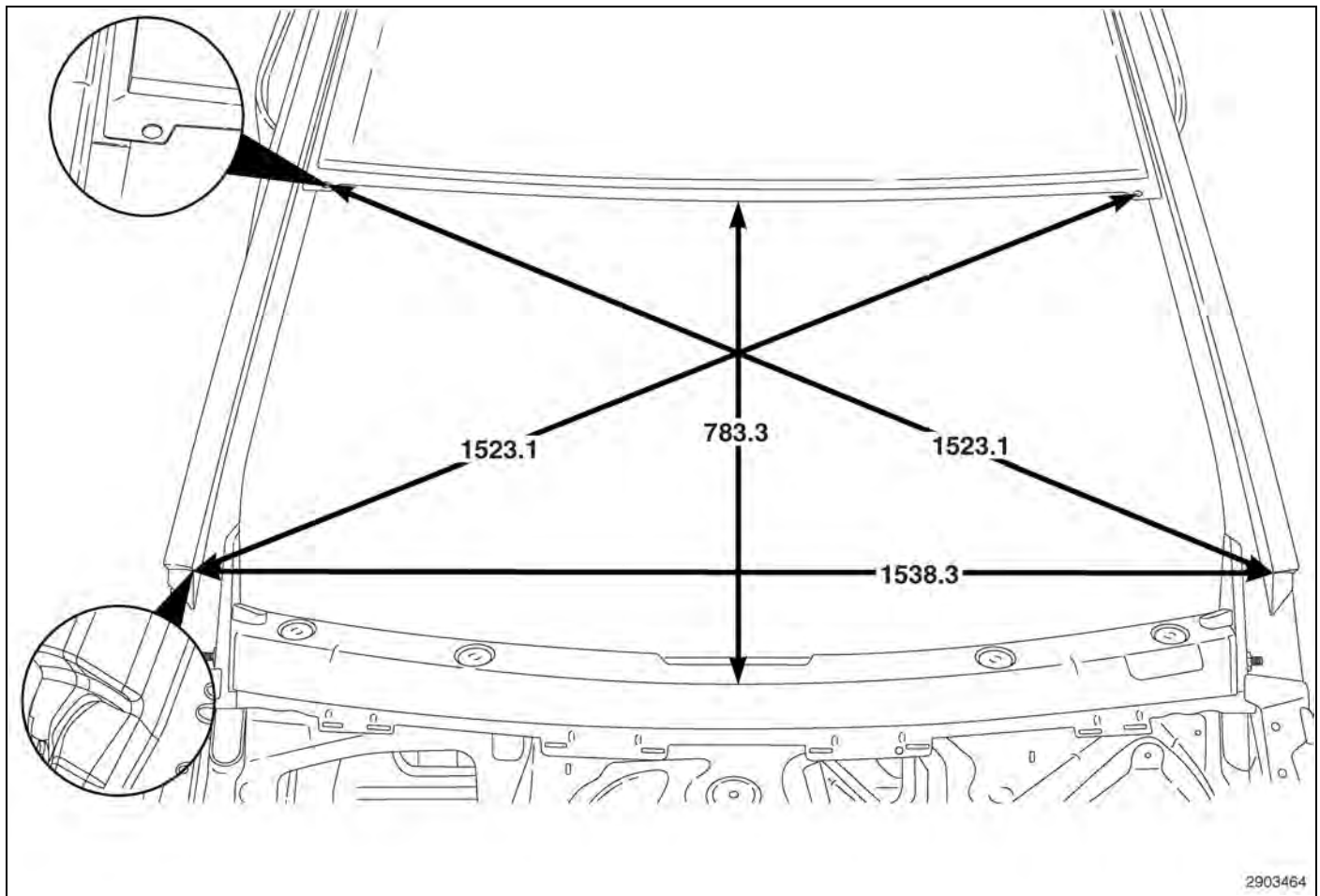
Fig. 1 Windshield
