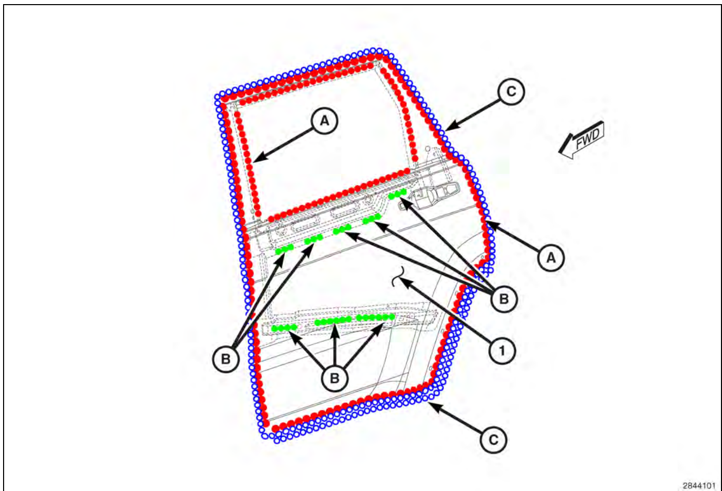
Fig. 51 Rear Door Shell
