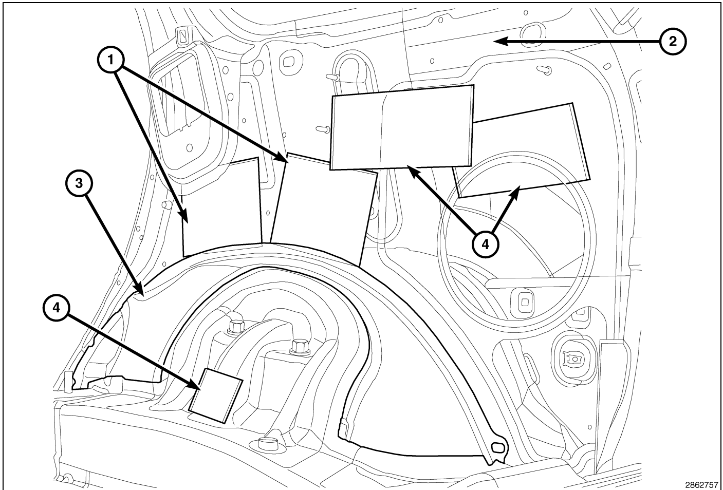
Fig. 44 Inner Body Side
