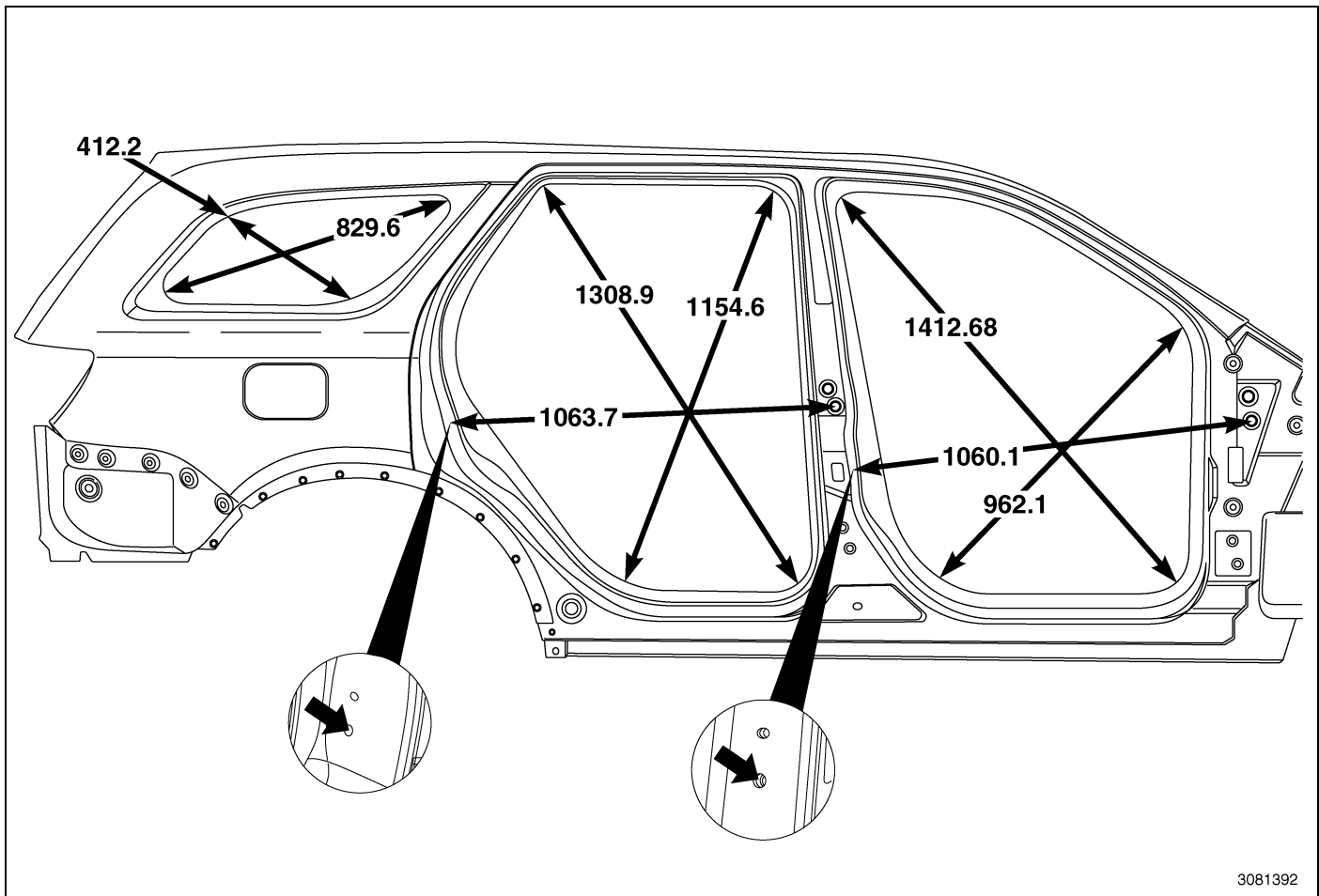
Fig. 2 Body Side Aperture
