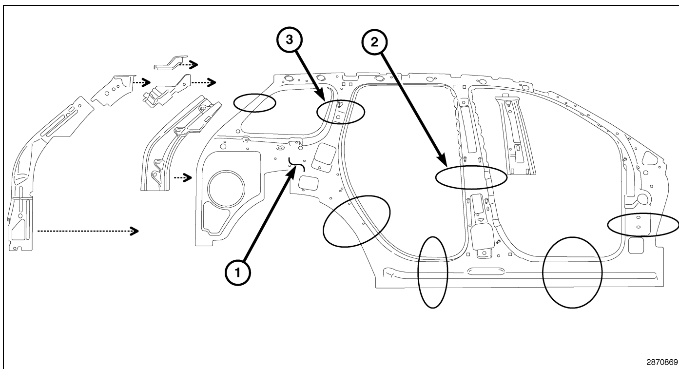
Fig. 23 Body Side Inner
