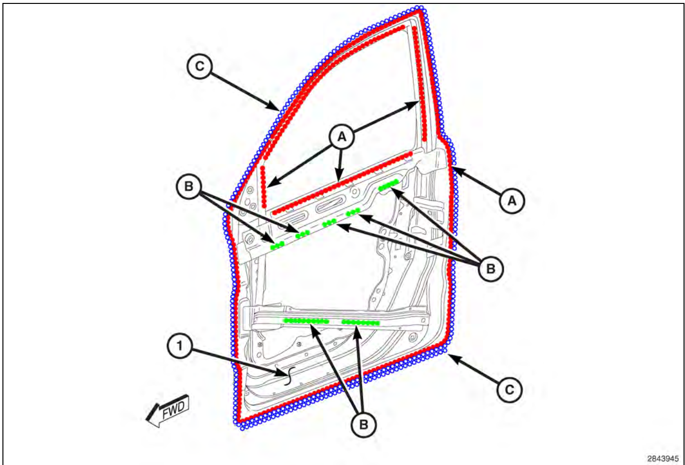
Fig. 50 Front Door Shell
